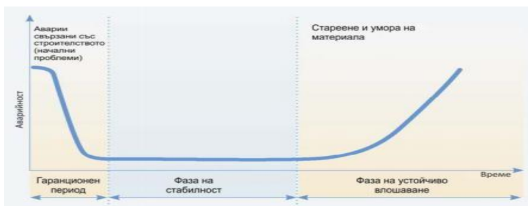
Фигура 2. Аварийност на тръбопроводите на водоснабдителната противопожарна мрежа
